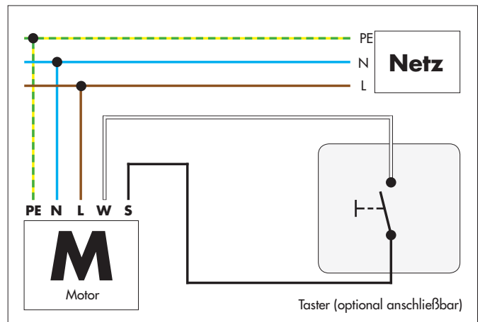
Abb.2: Anschlussschema Art. 140010 - 140050
